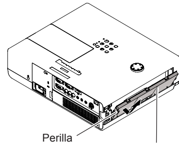
Perilla Unidades de filtro de aire (lateral)
