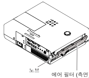
에어 필터 덮개 (측면)
