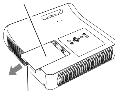
Крышка отсека лампы Винты крепления
