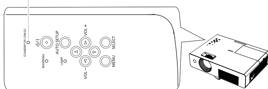
Spia STANDBY(R)/ON(G)
