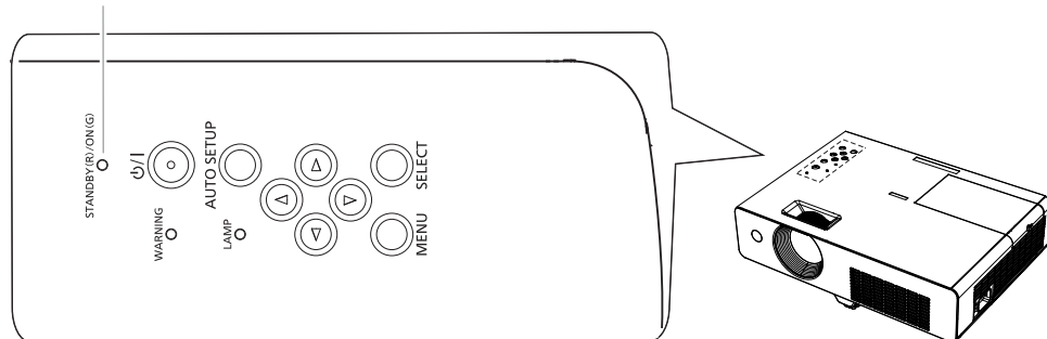
Индикатор STANDBY(R)/ON(G)
