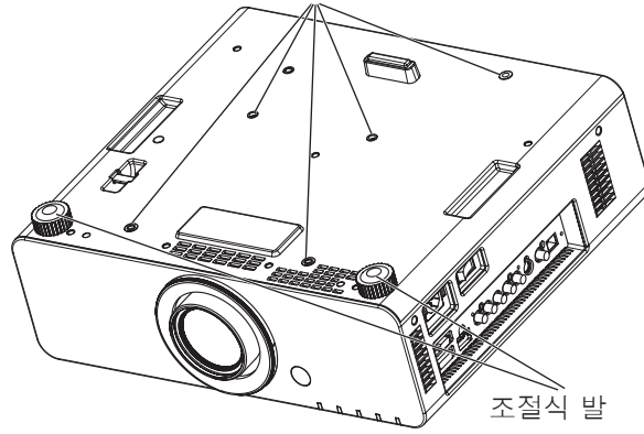
그림 1 천장 설치 및 조절식 발을 위한 나사 구멍 위치
