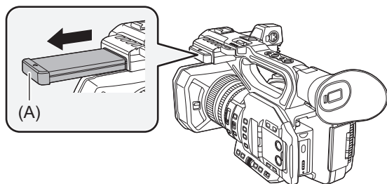
(A) Извлекатель ЖК-монитора
