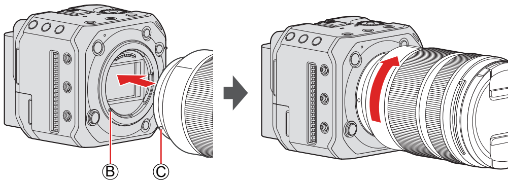
Ⓑ 镜头锁定销 Ⓒ 镜头安装标记
