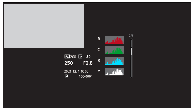
Histogram display
