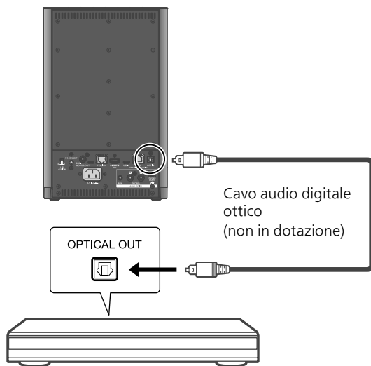
Dispositivo di uscita audio digitale
